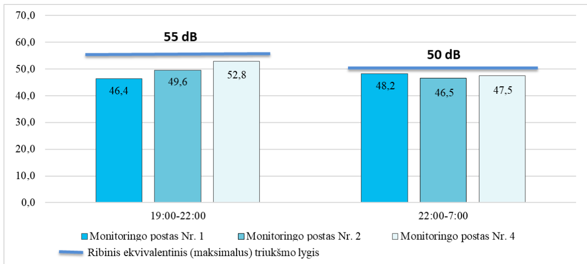
6 pav. UAB „NEO GROUP“ maksimalaus triukšmo matavimai monitoringo postuose
