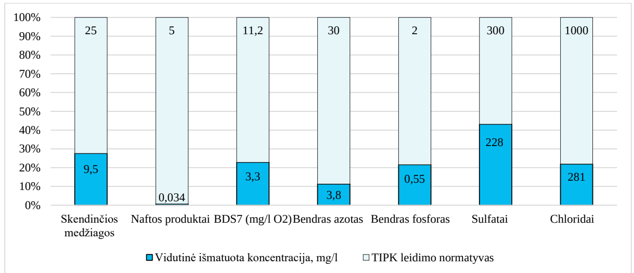
4 pav. UAB „NEO GROUP“ paviršinių nuotekų, išleidžiamų į melioracijos griovį, vidutinis užterštumas 2022 m.
