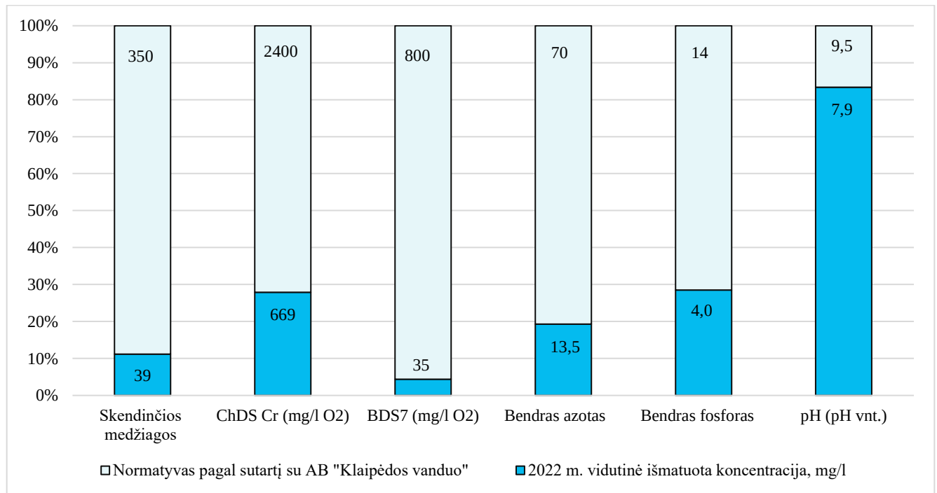
3 pav. UAB „NEO GROUP“ gamybinių - buitinių nuotekų, išleidžiamų į AB „Klaipėdos vanduo“ tinklus, užterštumas 2022 m.
