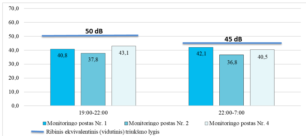
5 pav. UAB „NEO GROUP“ ekvivalentinio triukšmo matavimai monitoringo postuose
